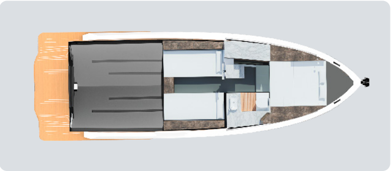
Distribución interior intraborda.
